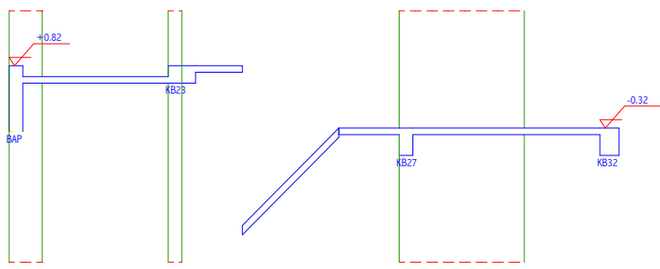
A-A kesiti (1/50)
